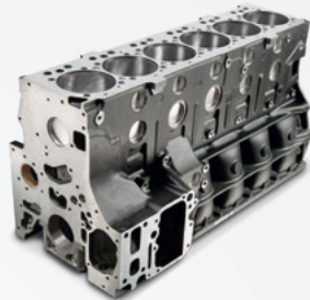
Kurbelgehäuse
